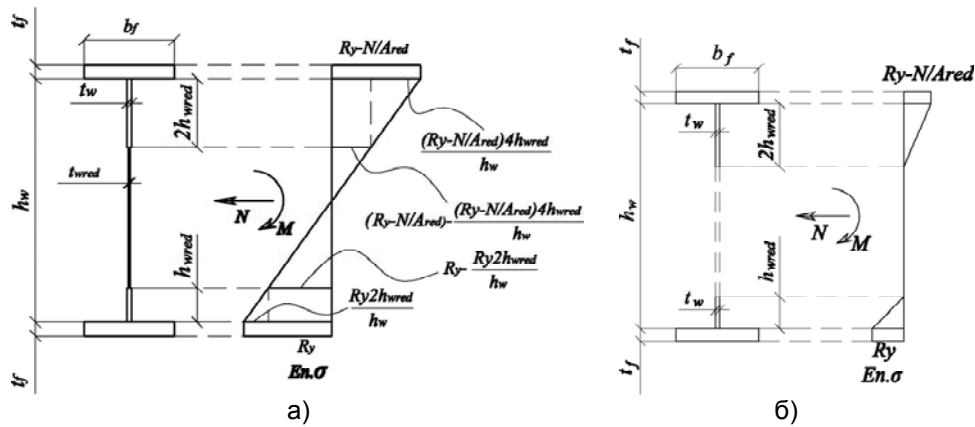
Рис. 4. а) розрахунковий переріз рами з гнучкою стінкою з урахуванням роботи стінки та з виключенням її з роботи; б) епюра нормальних напружень в перерізі.
